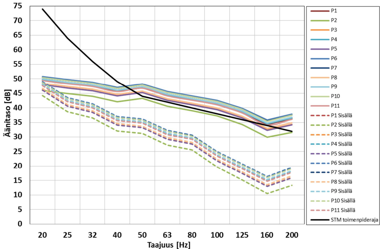
Kuva 4. Pientaajuisen melun laskentatulokset yhdeksässä lähimmässä reseptoripisteessä. Tulokäyrät asettuvat osin lähes päällekkäin laskentatulosten samankaltaisuuksien vuoksi.
